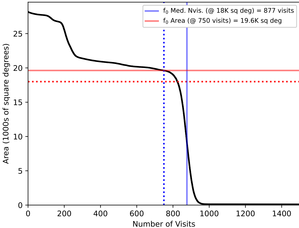
weather_cloudso6v3.5_10yrs : fO
