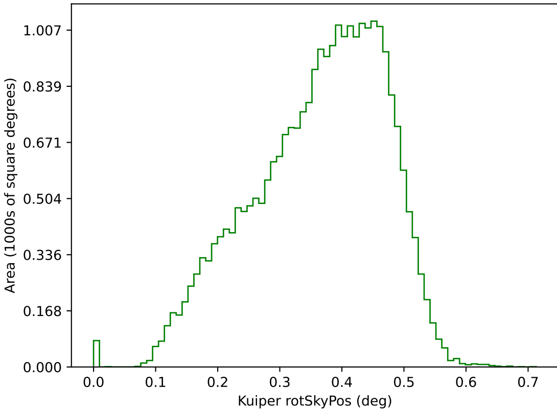
weather_cloudso6v3.5_10yrs g: Kuiper rotSkyPos
