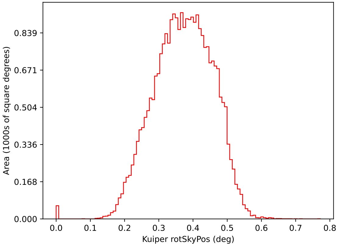
weather_cloudso6v3.5_10yrs i: Kuiper rotSkyPos
