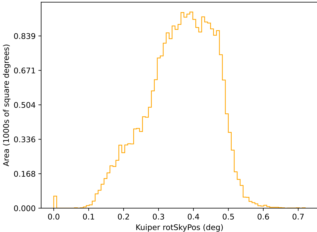
weather_cloudso6v3.5_10yrs r: Kuiper rotSkyPos
