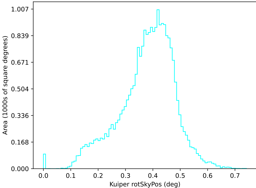
weather_cloudso6v3.5_10yrs u: Kuiper rotSkyPos
