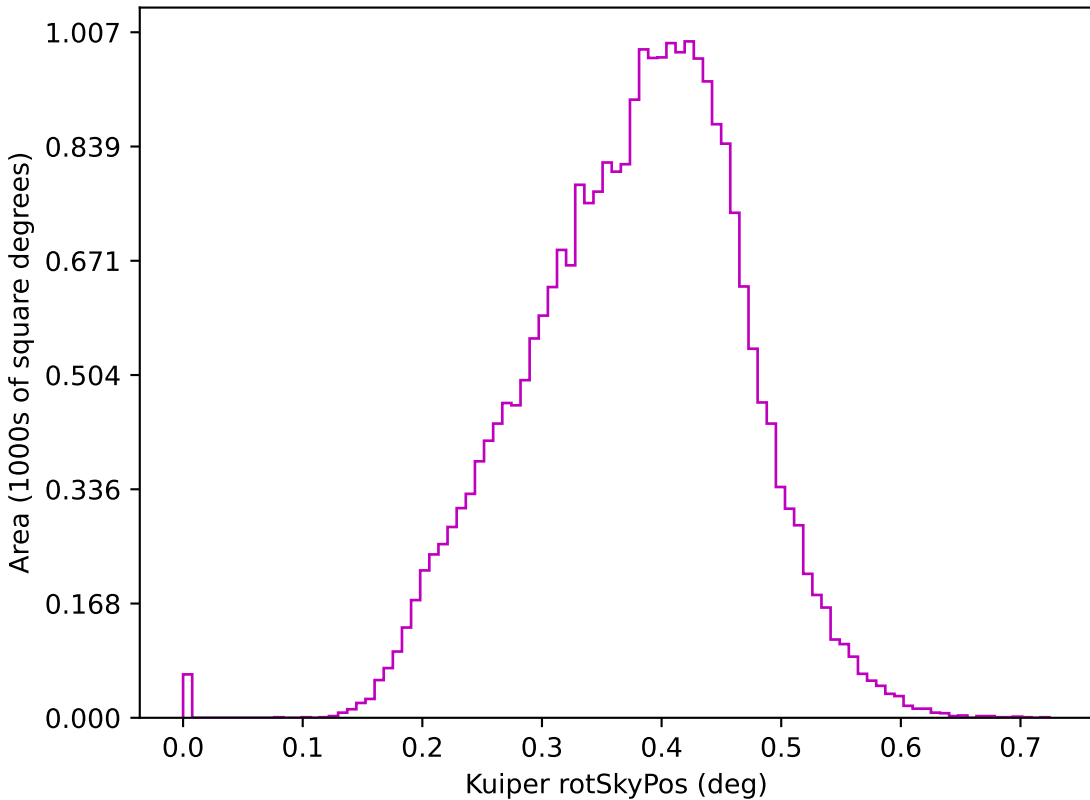
weather_cloudso6v3.5_10yrs z: Kuiper rotSkyPos
