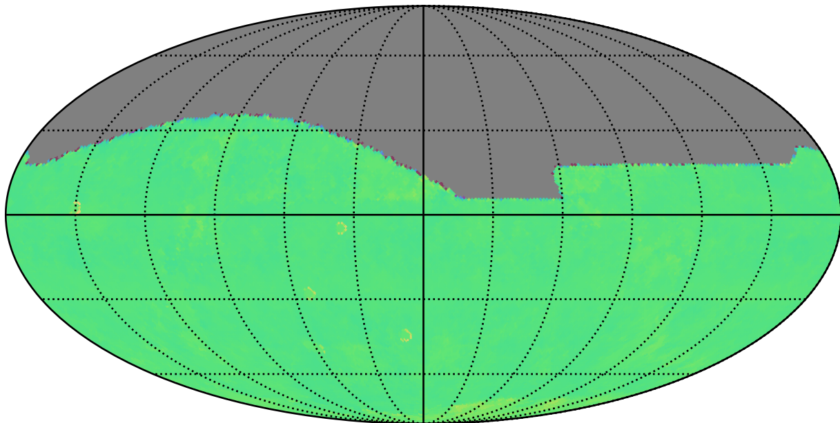
weather_cloudso6v3.5_10yrs r: Kuiper rotTelPos
