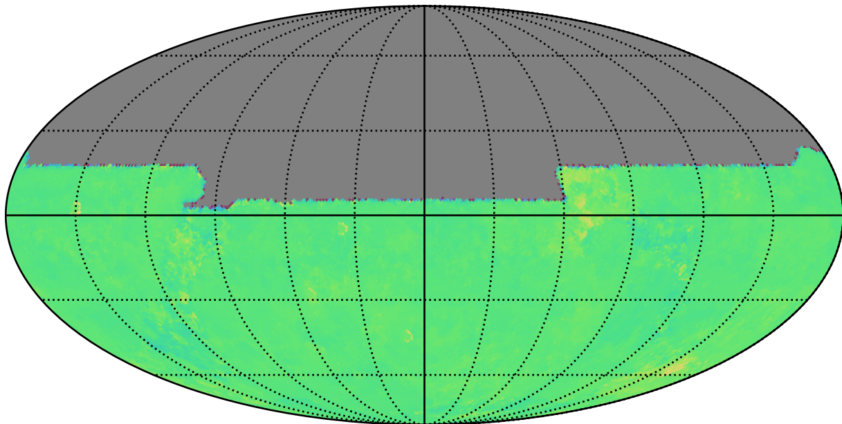
weather_cloudso6v3.5_10yrs u: Kuiper rotTelPos
