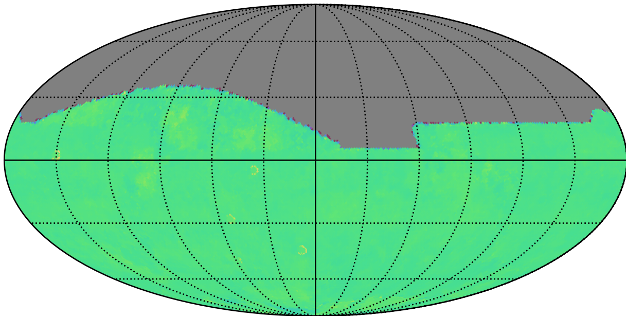
weather_cloudso6v3.5_10yrs z: Kuiper rotTelPos
