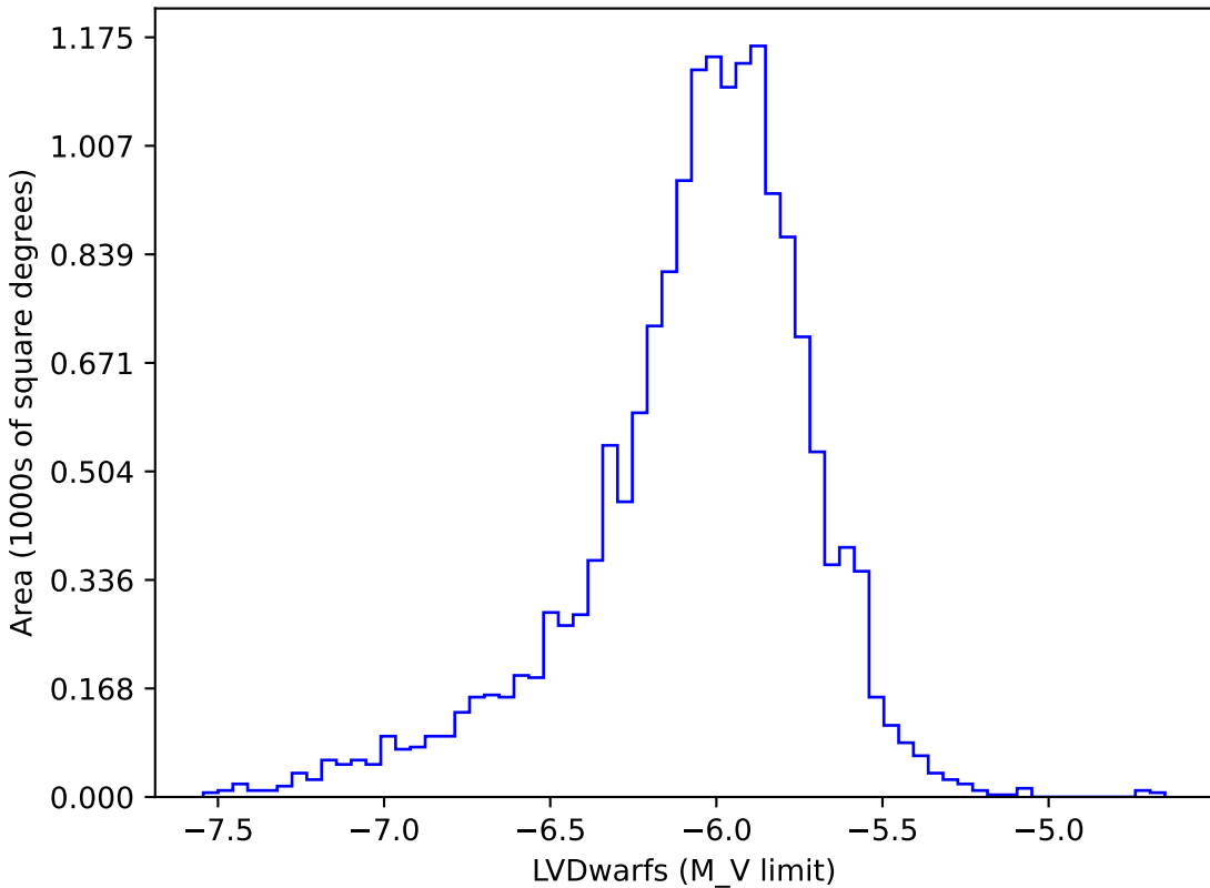
weather_cloudso6v3.5_10yrs gi: LVDwarfs
