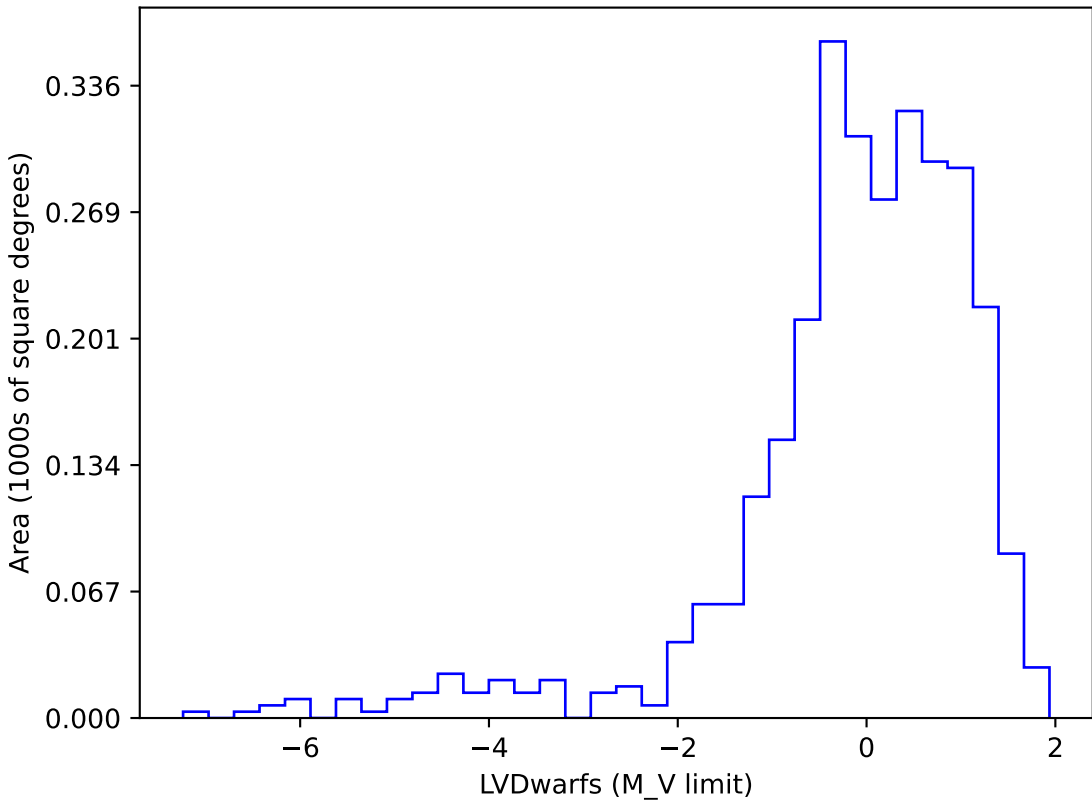
weather_cloudso6v3.5_10yrs gi SCP: LVDwarfs
