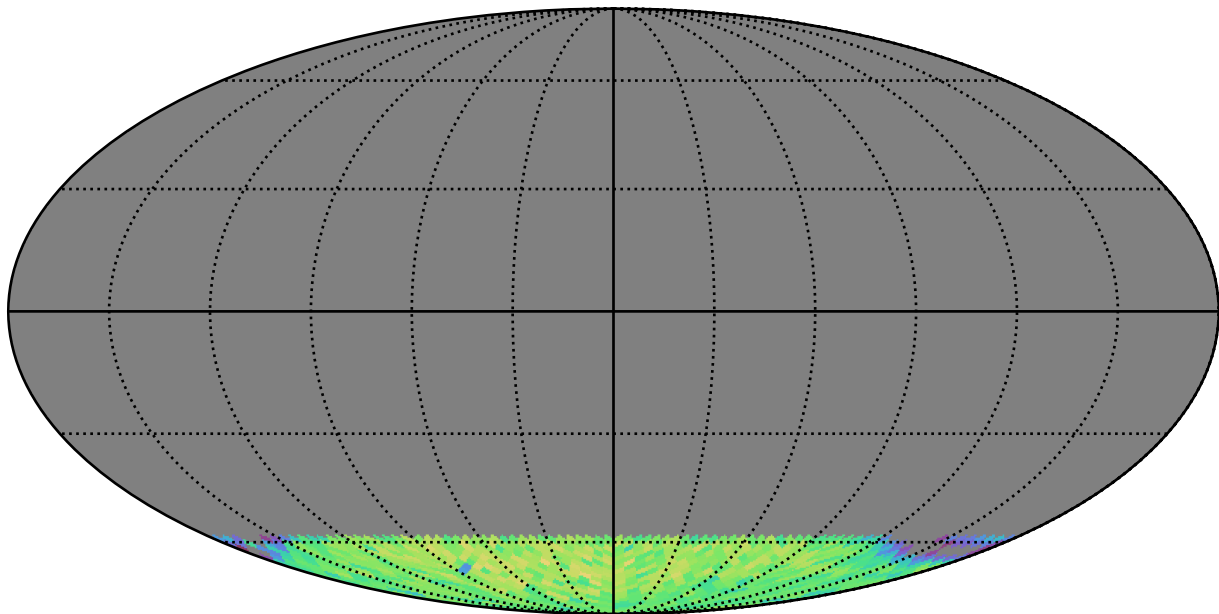
weather_cloudso6v3.5_10yrs gi SCP: LVDwarfs
