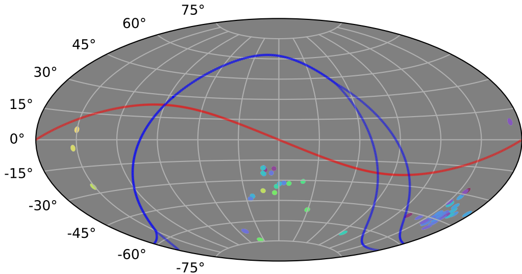
weather_cloudso6v3.5_10yrs gi: LVDwarfs
