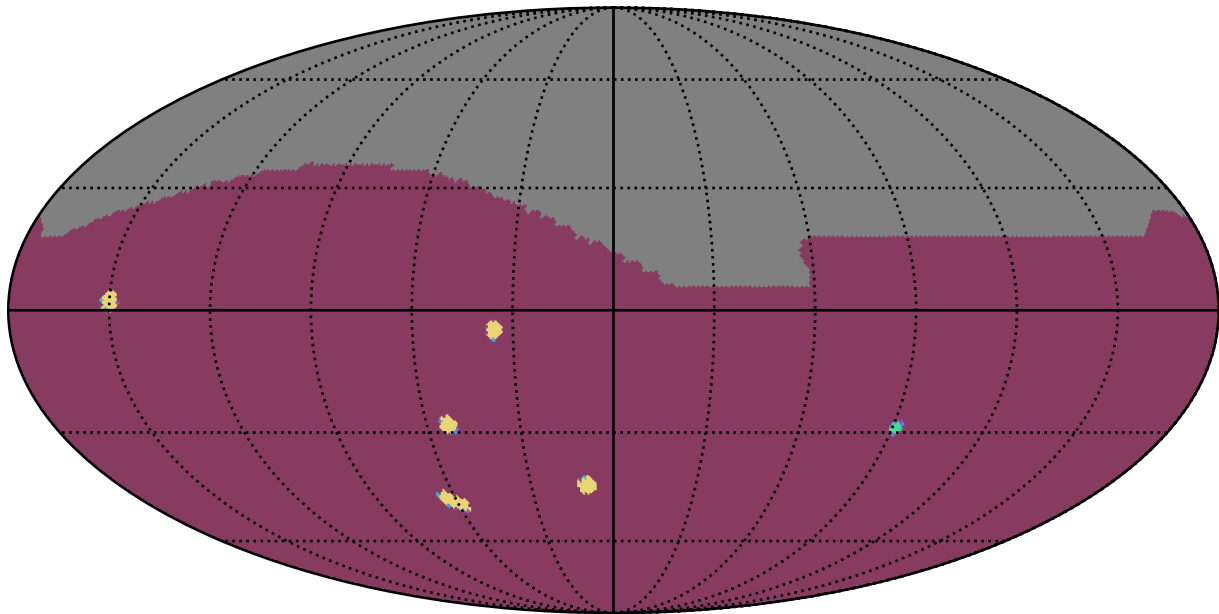
weather_cloudso6v3.5_10yrs : NumberOfQuickRevisits
