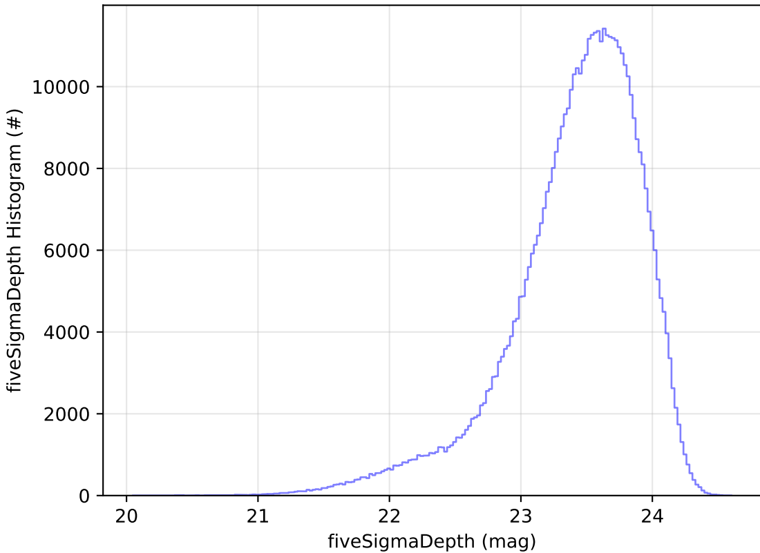
weather_cloudso6v3.5_10yrs i: fiveSigmaDepth Histogram
