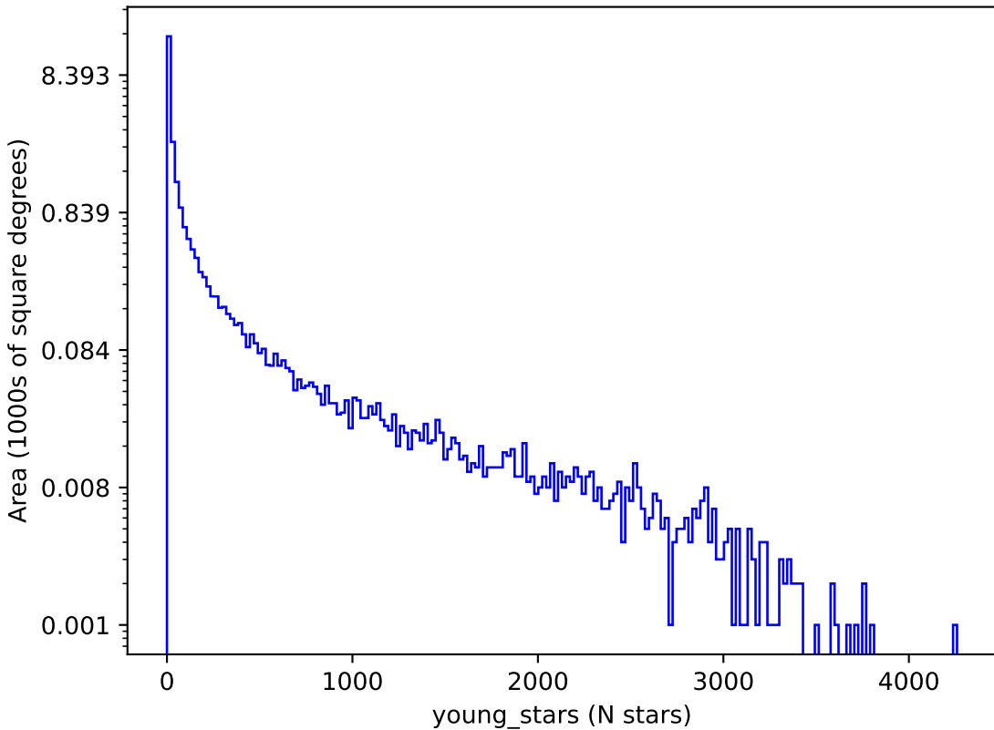
weather_cloudso6v3.5_10yrs : young_stars
