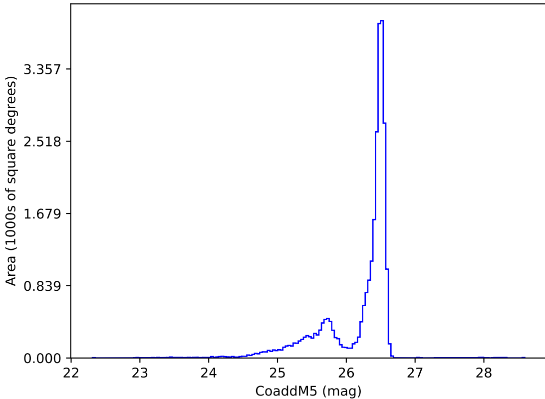
weather_cloudso8v3.5_10yrs i: CoaddM5
