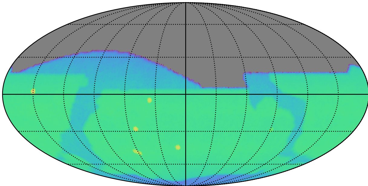
weather_cloudso8v3.5_10yrs i: CoaddM5
