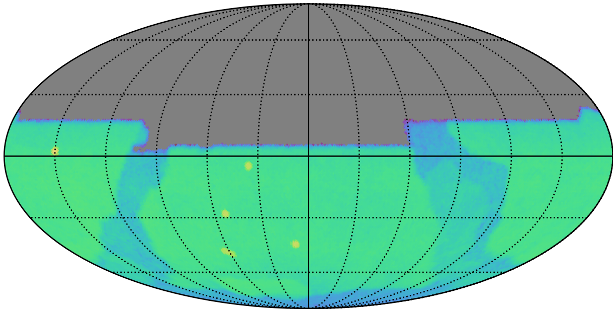
weather_cloudso8v3.5_10yrs u: CoaddM5
