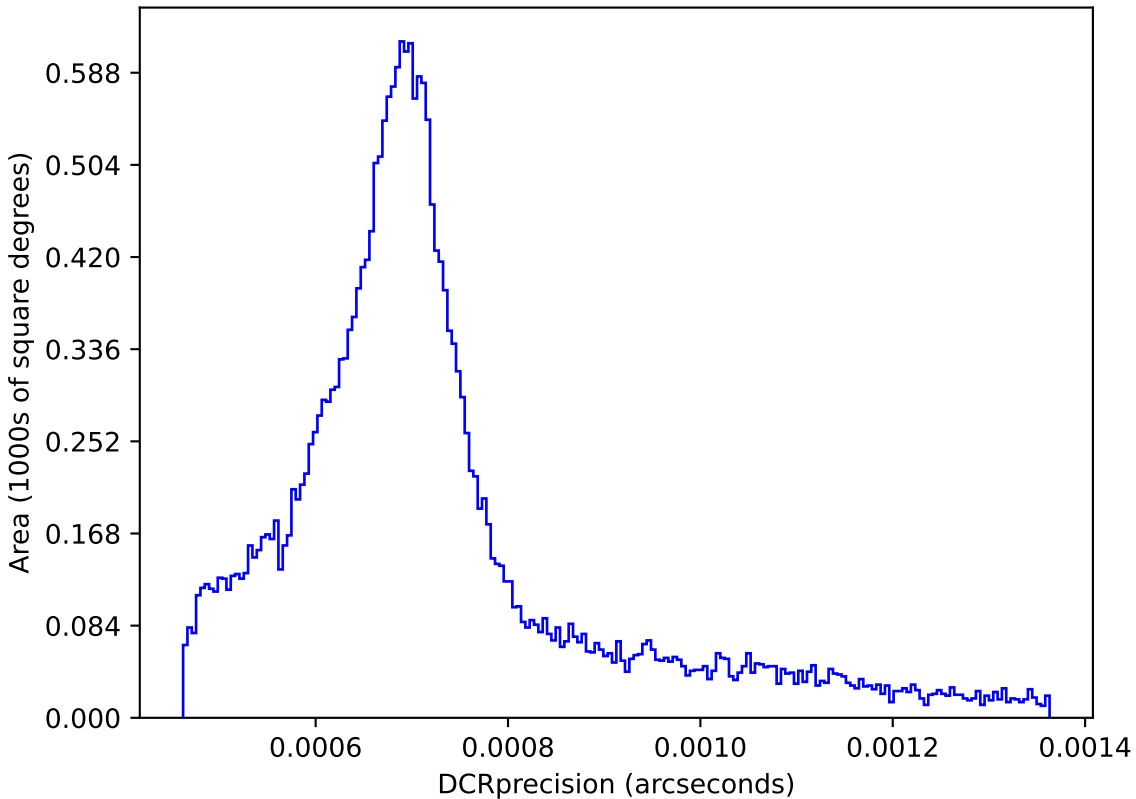
weather_cloudso8v3.5_10yrs : DCRprecision
