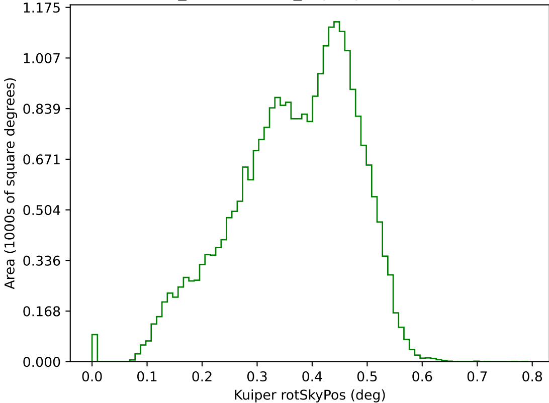
weather_cloudso8v3.5_10yrs g: Kuiper rotSkyPos
