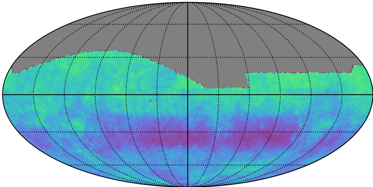
weather_cloudso8v3.5_10yrs g: Kuiper rotSkyPos
