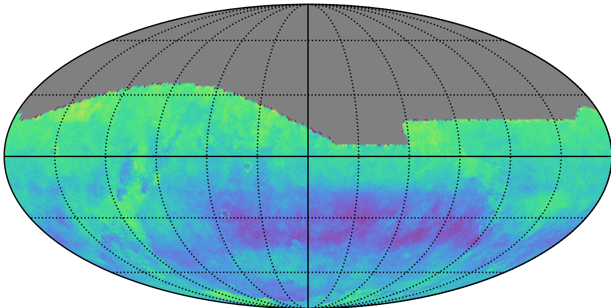
weather_cloudso8v3.5_10yrs i: Kuiper rotSkyPos
