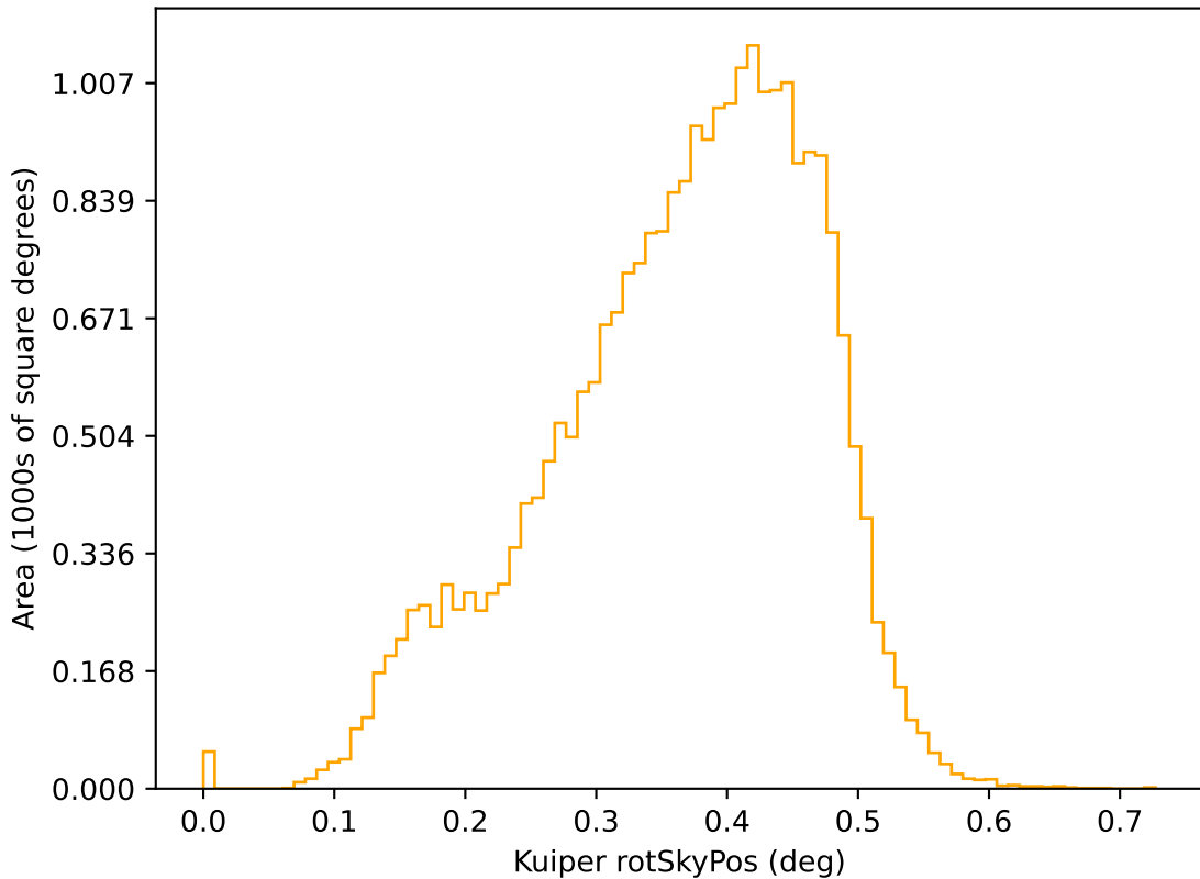
weather_cloudso8v3.5_10yrs r: Kuiper rotSkyPos
