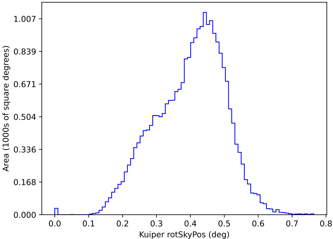
weather_cloudso8v3.5_10yrs y: Kuiper rotSkyPos
