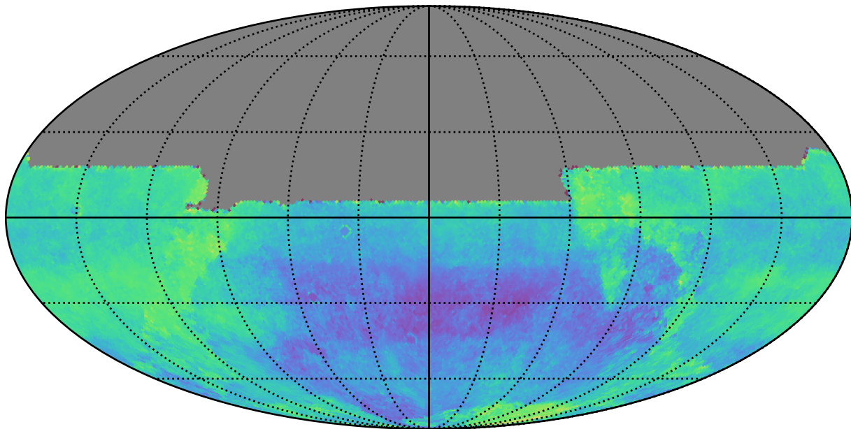
weather_cloudso8v3.5_10yrs y: Kuiper rotSkyPos
