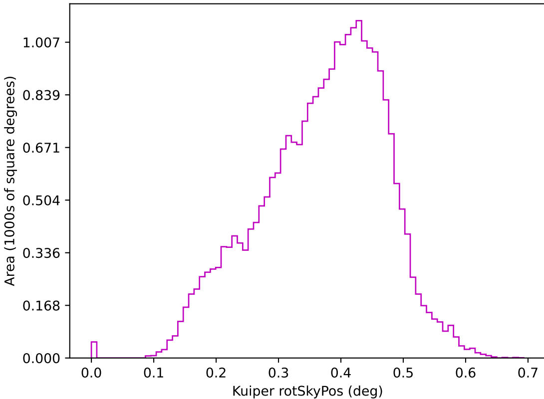
weather_cloudso8v3.5_10yrs z: Kuiper rotSkyPos
