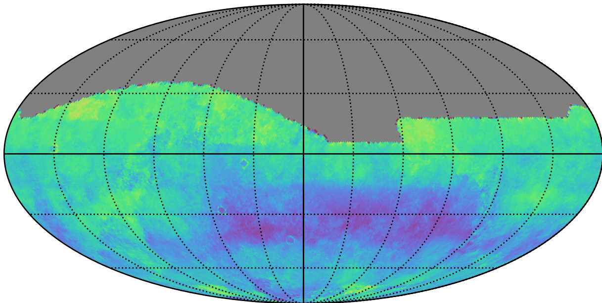
weather_cloudso8v3.5_10yrs z: Kuiper rotSkyPos
