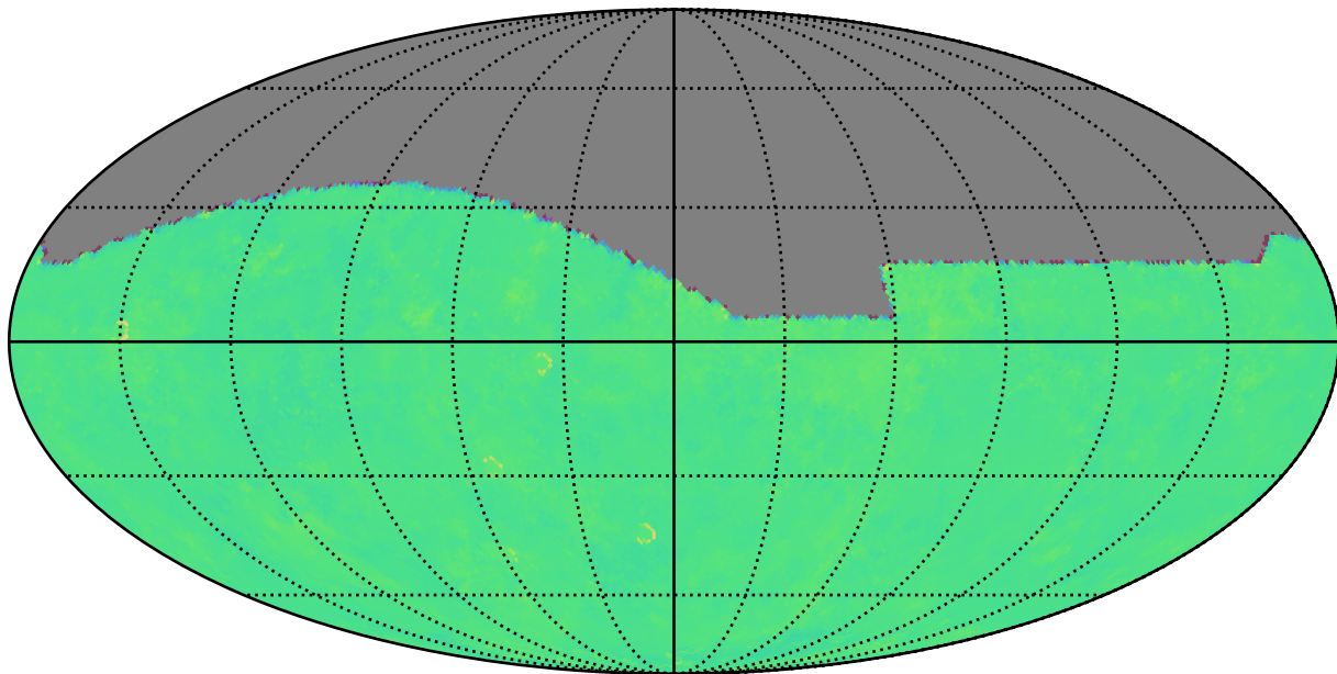
weather_cloudso8v3.5_10yrs g: Kuiper rotTelPos
