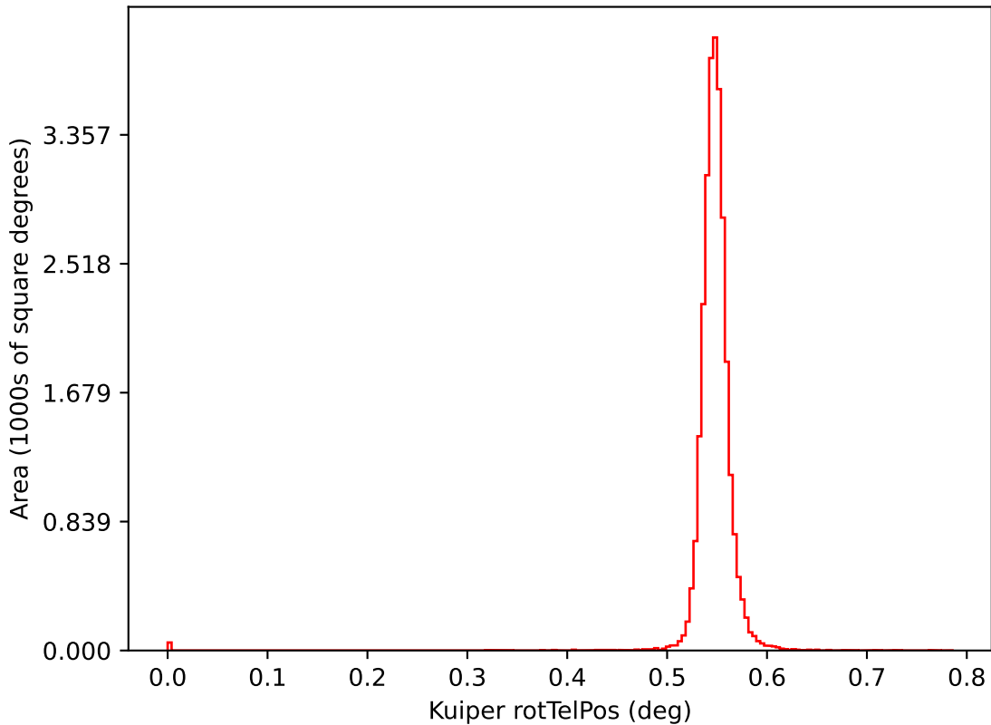
weather_cloudso8v3.5_10yrs i: Kuiper rotTelPos
