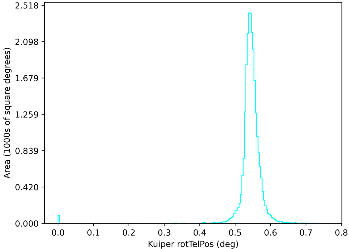
weather_cloudso8v3.5_10yrs u: Kuiper rotTelPos
