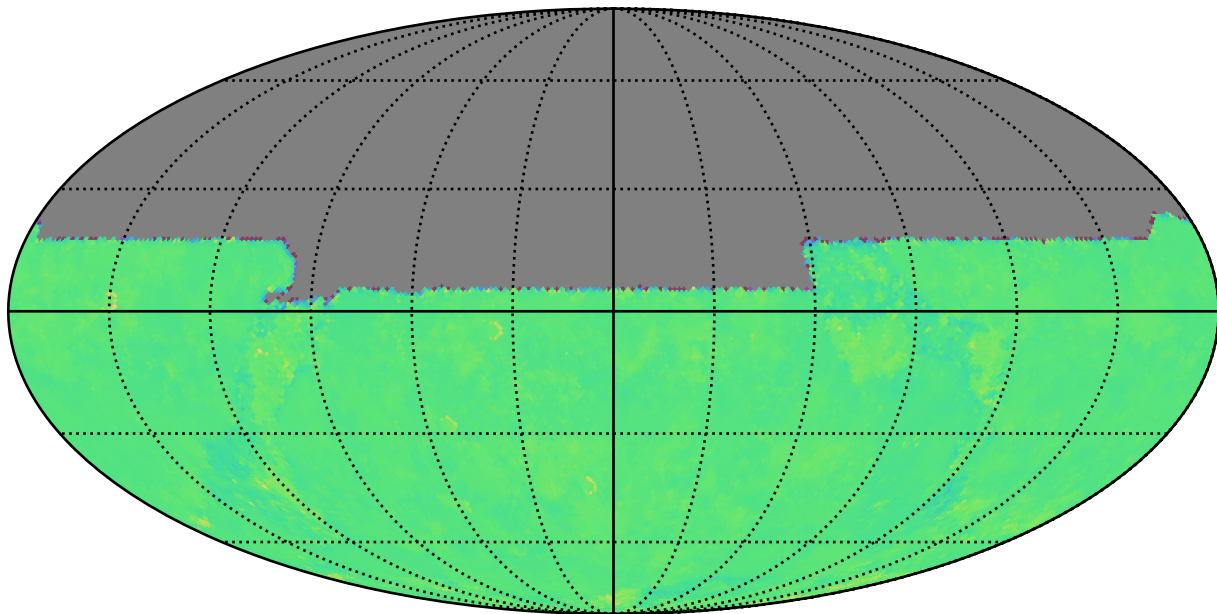
weather_cloudso8v3.5_10yrs u: Kuiper rotTelPos
