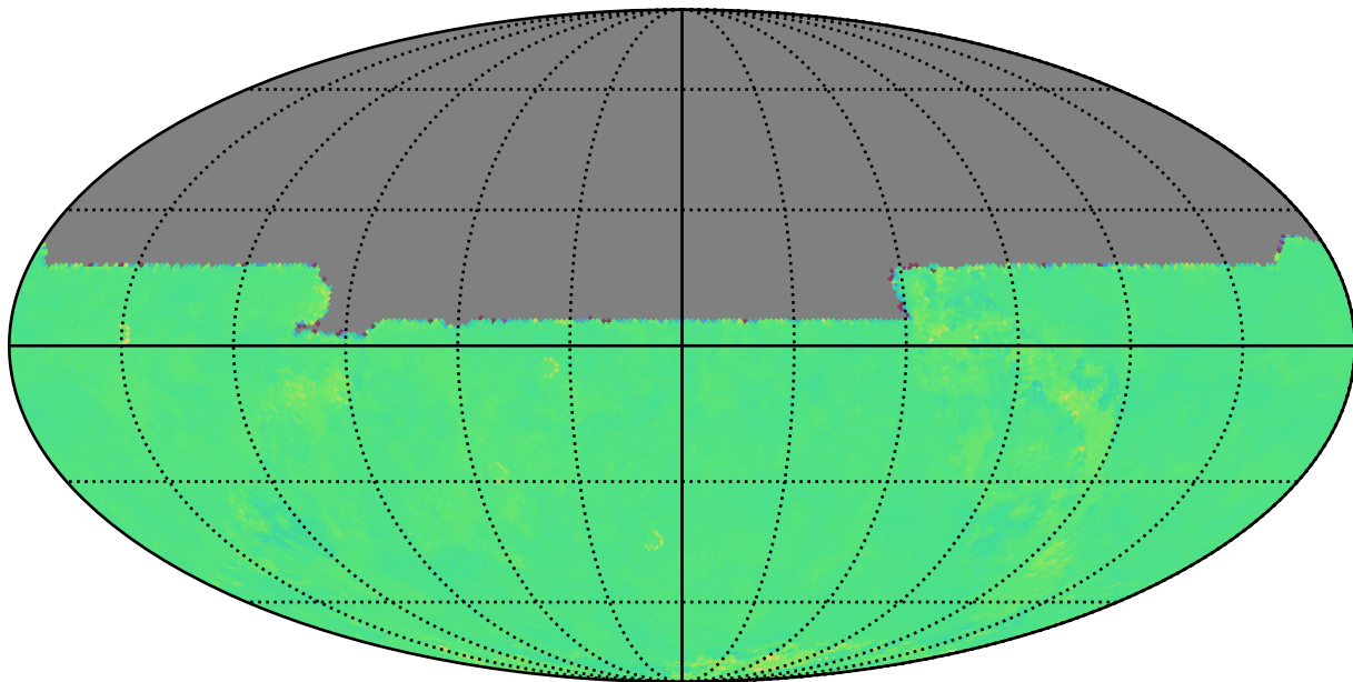
weather_cloudso8v3.5_10yrs y: Kuiper rotTelPos
