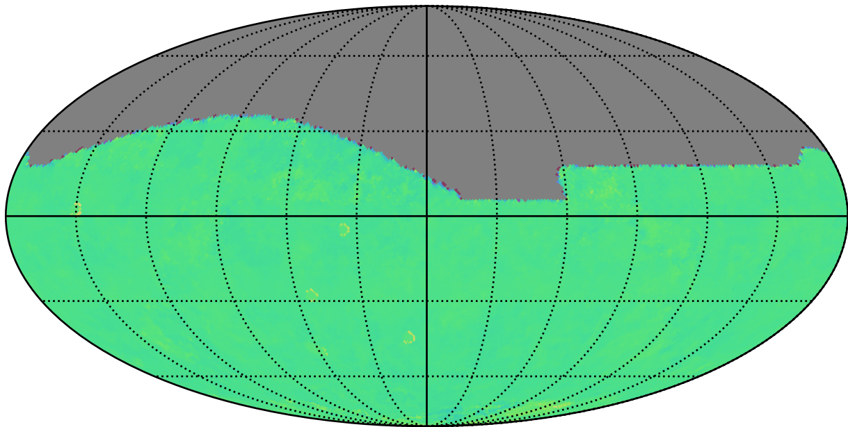
weather_cloudso8v3.5_10yrs z: Kuiper rotTelPos
