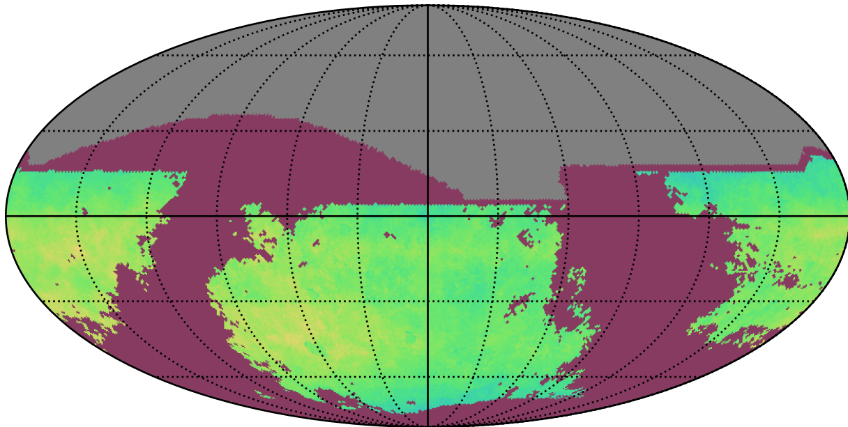
weather_cloudso8v3.5_10yrs i: NgalScale
