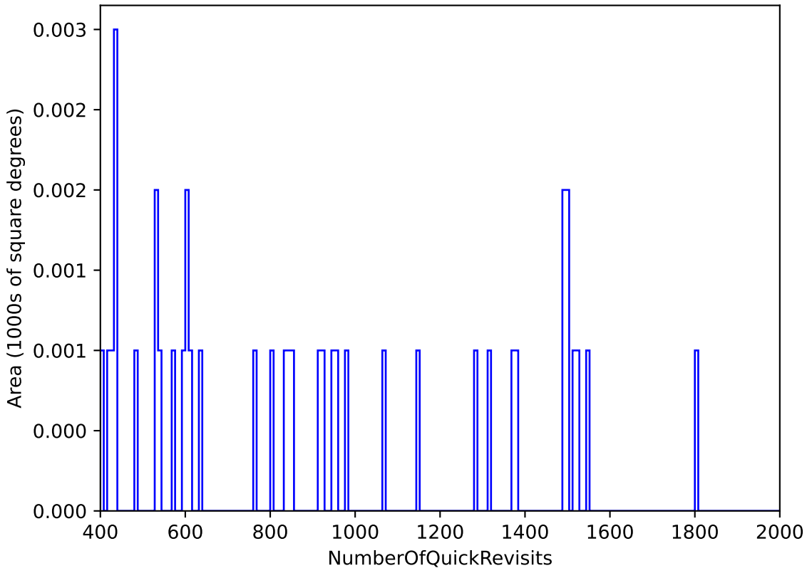
weather_cloudso8v3.5_10yrs : NumberOfQuickRevisits
