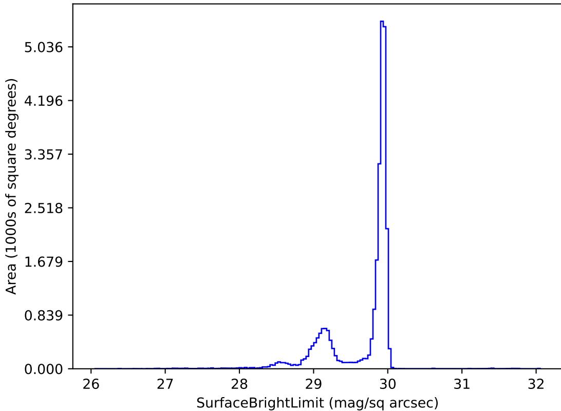
weather_cloudso8v3.5_10yrs i: SurfaceBrightLimit
