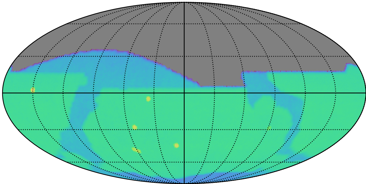
weather_cloudso8v3.5_10yrs i: SurfaceBrightLimit
